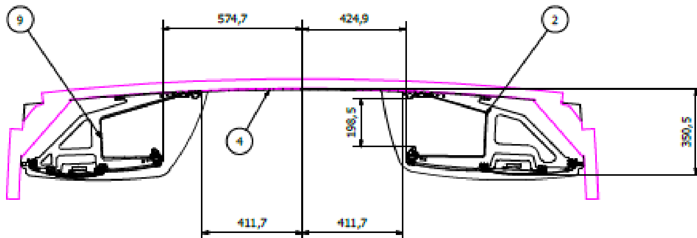
A-A ( 1:10 )
